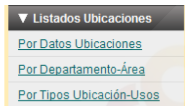
Figura 1.14. Hiperenlace.
